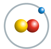
Deuterium atom
